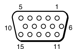
Toma D-sub de 15 patillas "shrink"
